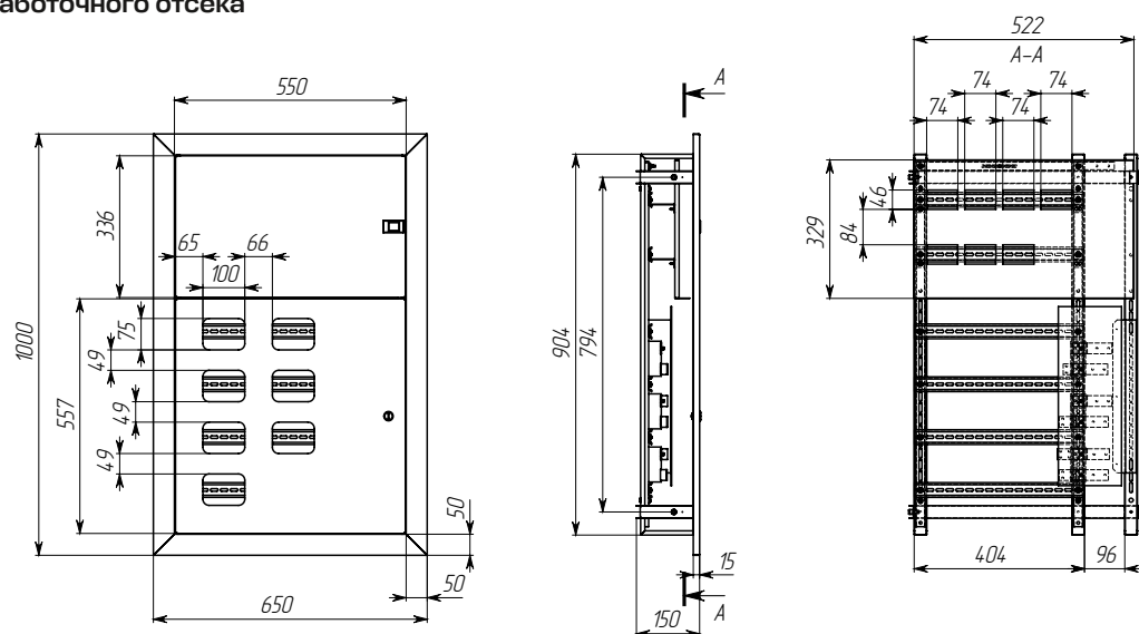
ЩЭ 7 кв. без слаботочного отсека
