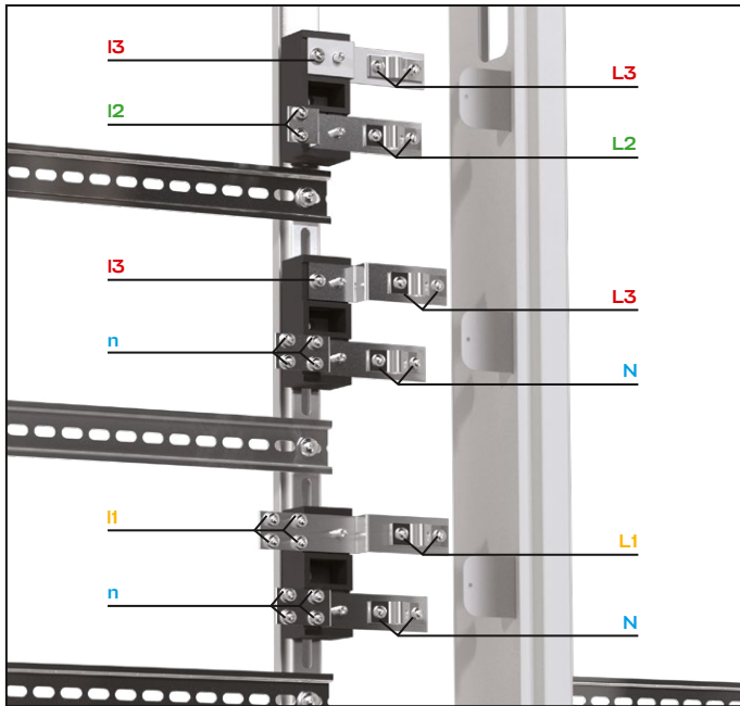
Обозначения: L1, L2, L3 – места крепления магистральных фазных кабелей, N – место крепления магистрального нейтрального кабеля, I1, I2, I3 – места крепления отходящих фазных кабелей, n – места крепления отходящих нейтральных кабелей.
