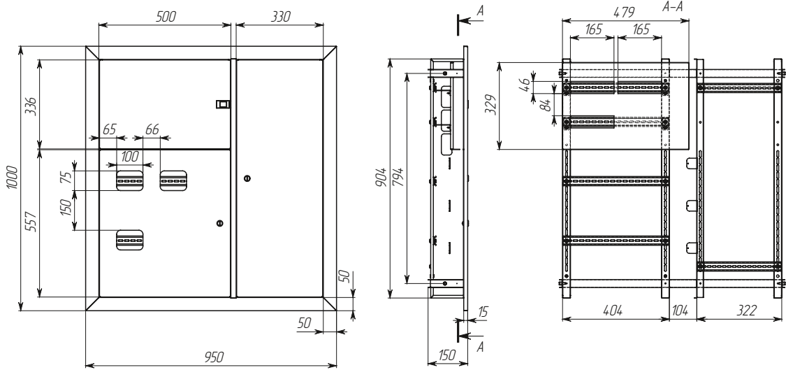
Щит этажный 3 кв.
