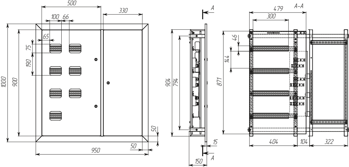
ЩЭ 7 кв. 2-дверный
