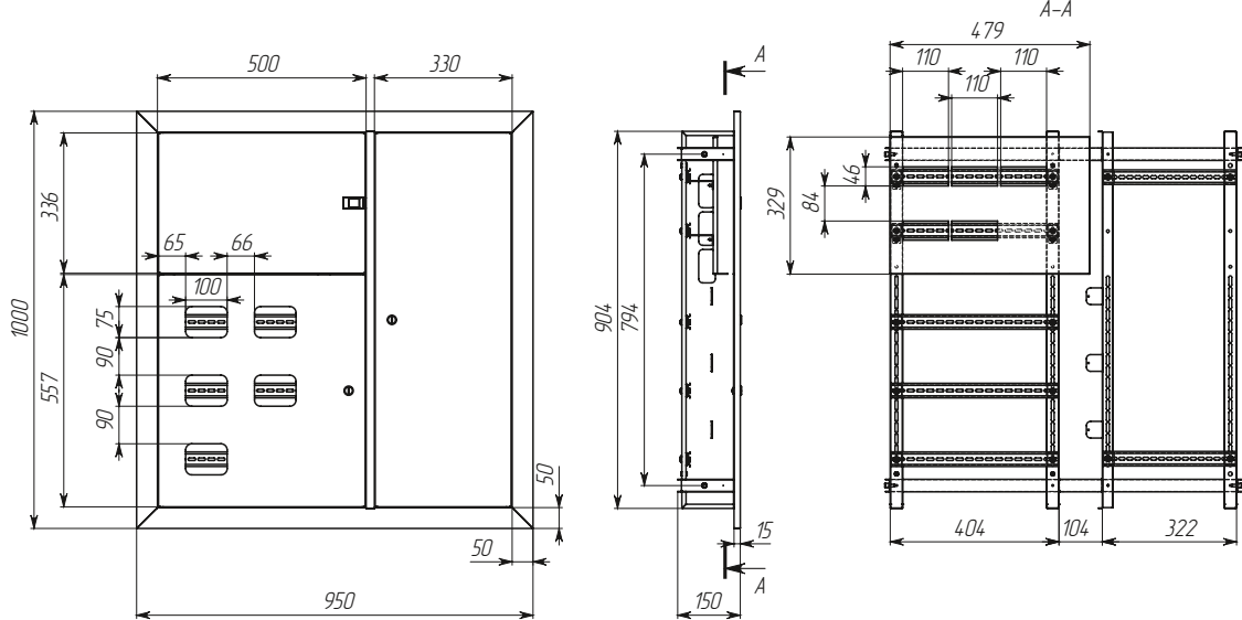
Щит этажный 5 кв.
