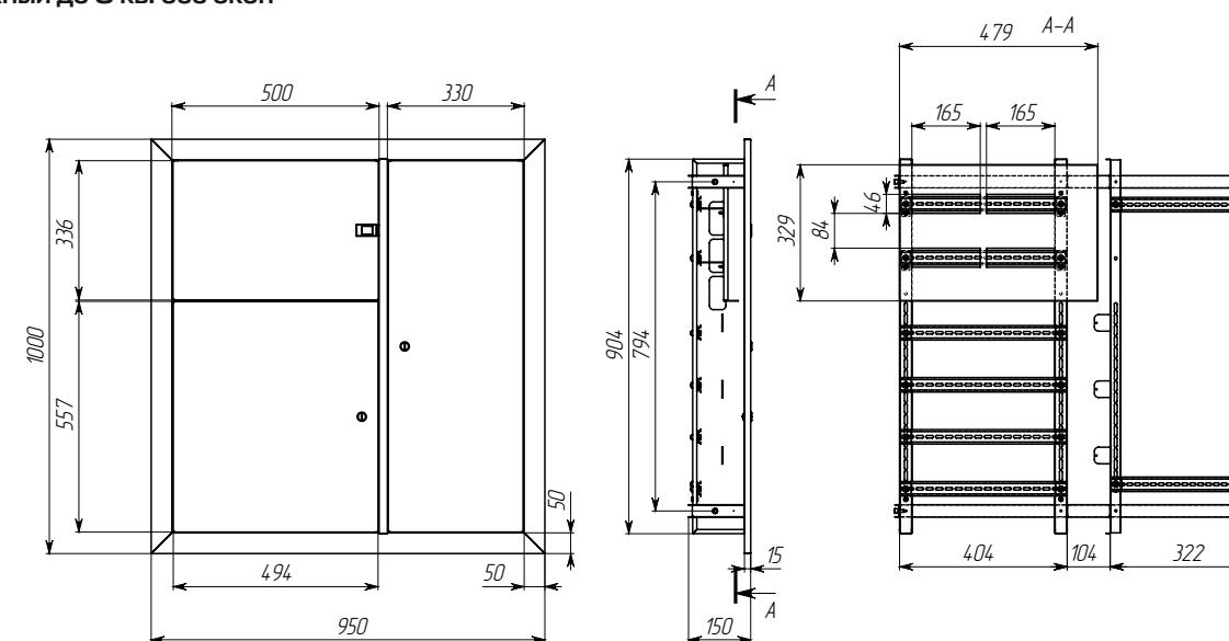
Щит этажный до 8 кв. без окон
