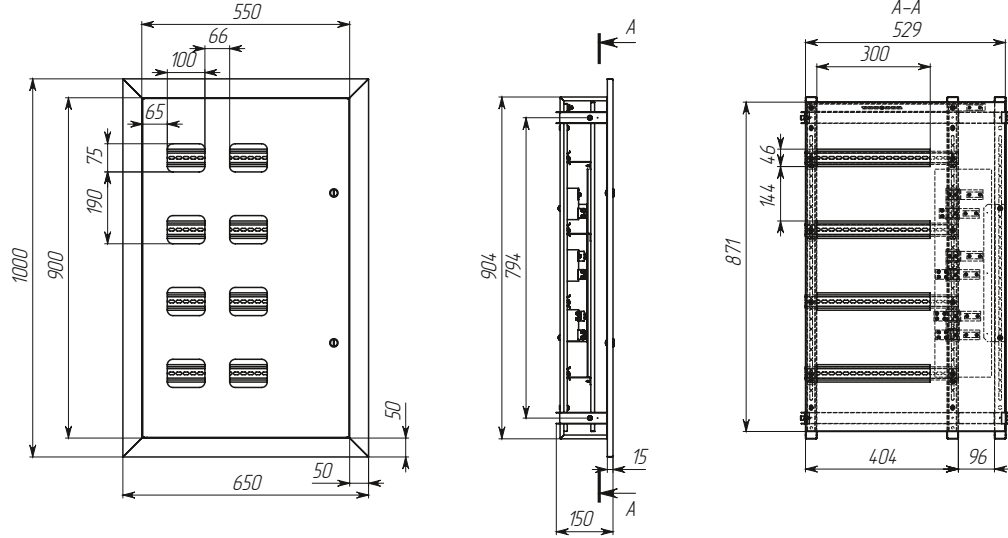
ЩЭ 9 кв. без слаботочного отсека 1-дверный
