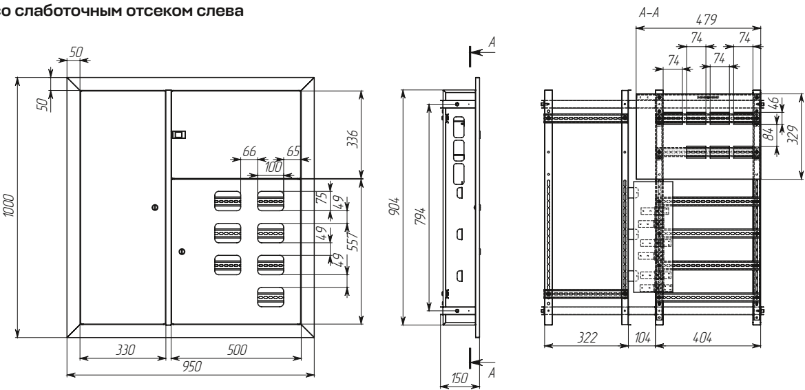
ЩЭ 8 кв. со слаботочным отсеком слева
