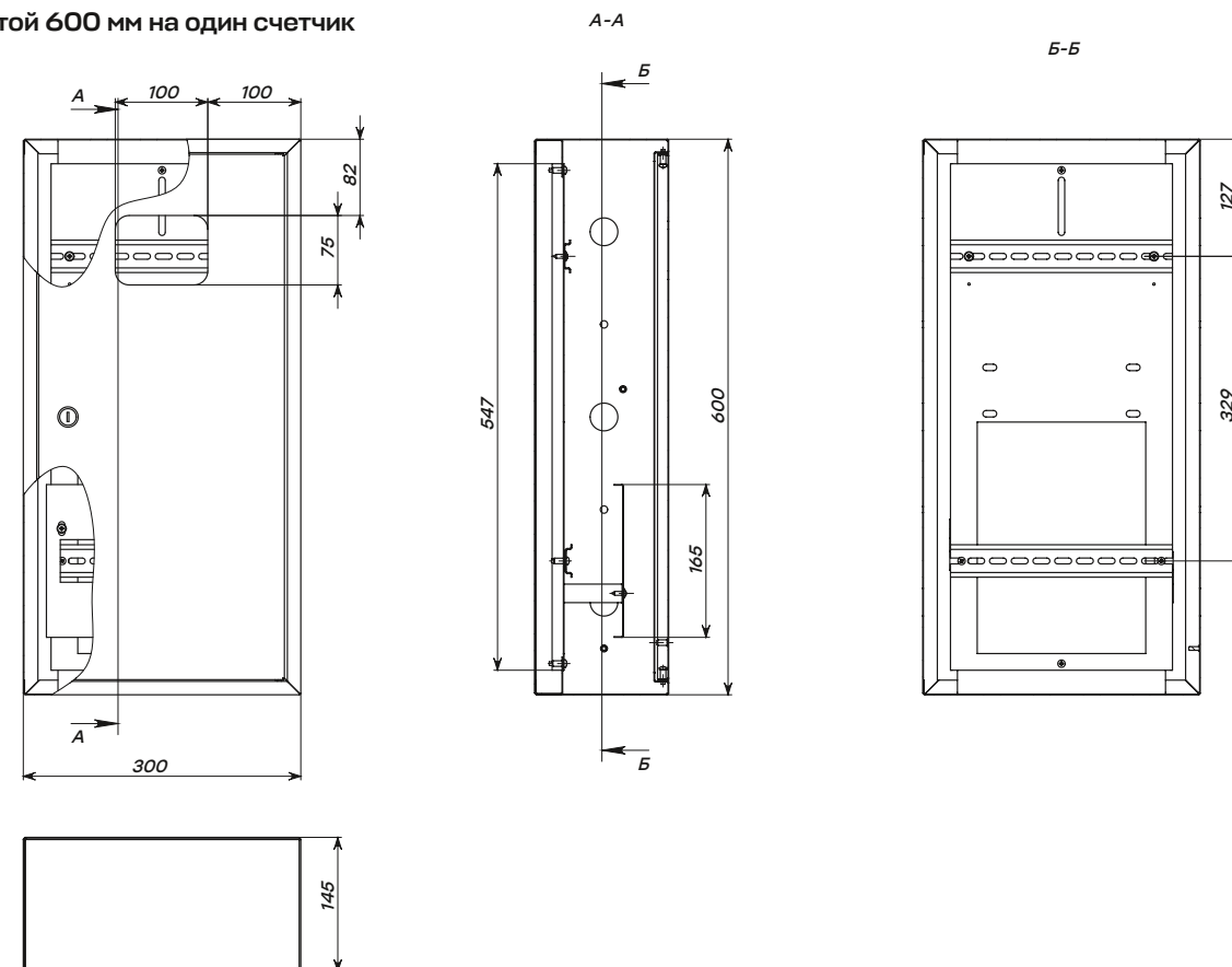
ЯУР высотой 600 мм на один счетчик
