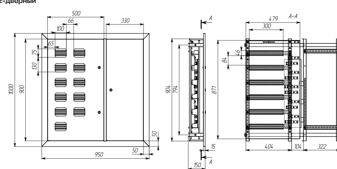
ЩЭ 12 кв. 2-дверный
