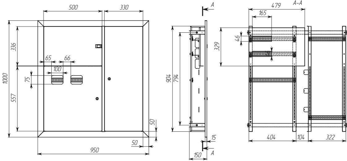
Щит этажный 2 кв.
