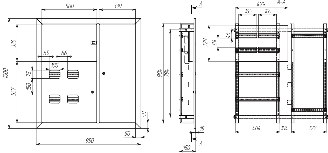
Щит этажный 4 кв.
