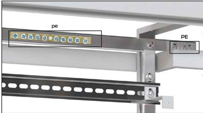
Обозначения: PE – место крепления магистрального кабеля заземления, pe – место крепления кабелей, отходящих в квартиры (где 1-8 – количество квартир).
