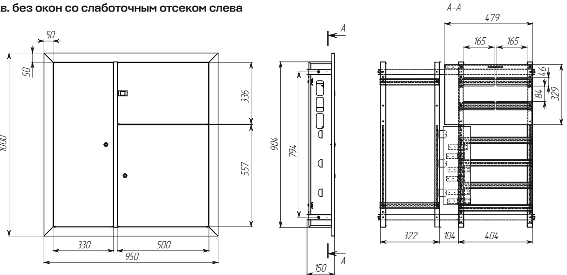
ЩЭ до 8 кв. без окон со слаботочным отсеком слева
